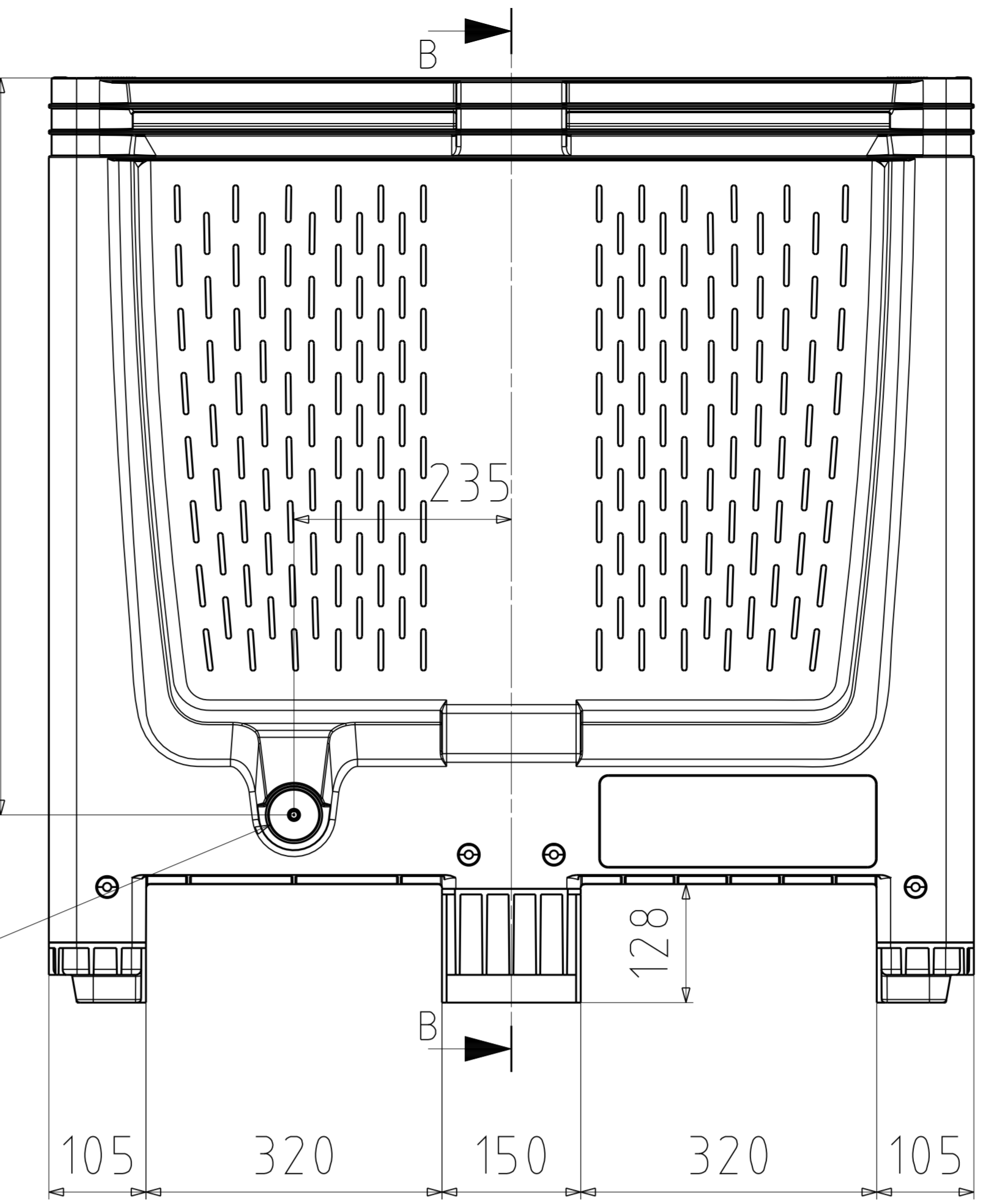
Schnitt B-B
